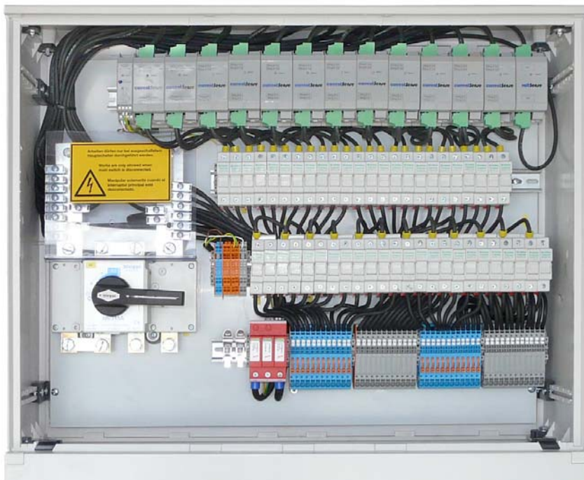
Ausführung mit Einzelstrangmessung
