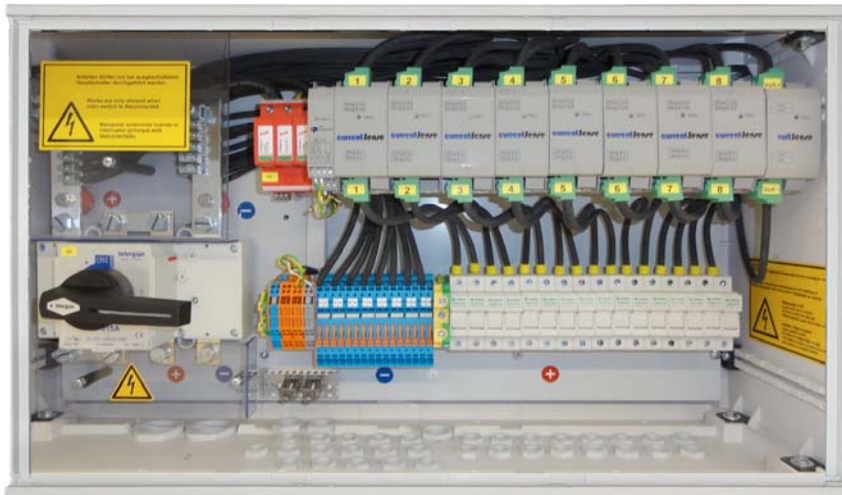
Gehäuse zur Wand- oder Gestellmontage (Schließzylinder optional)
